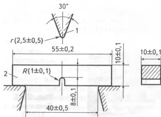
Рис. 2.16 Схема визначення ударної в'язкості: 1 — боек маятника; 2 — зразок
