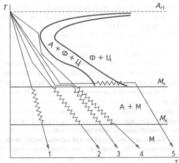
Рис. 4.25 Графіки режимів охолодження в процесі гартування:
