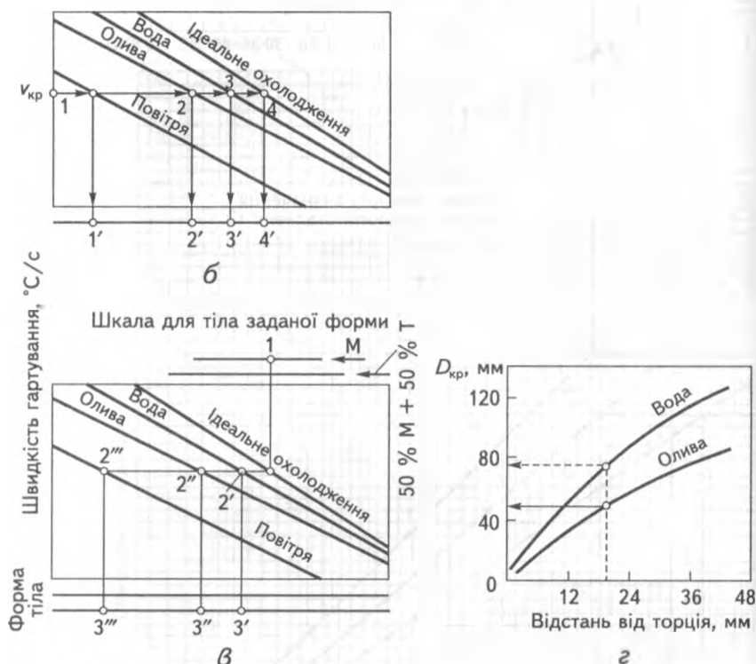
Рис. 4.20 Номограма для визначення прогартуваності сталевих тіл (а) (с. 142—143). Визначення прогартуваності за критичною швидкістю v_{кр} (б) і за торцевою пробєю (в, г)
