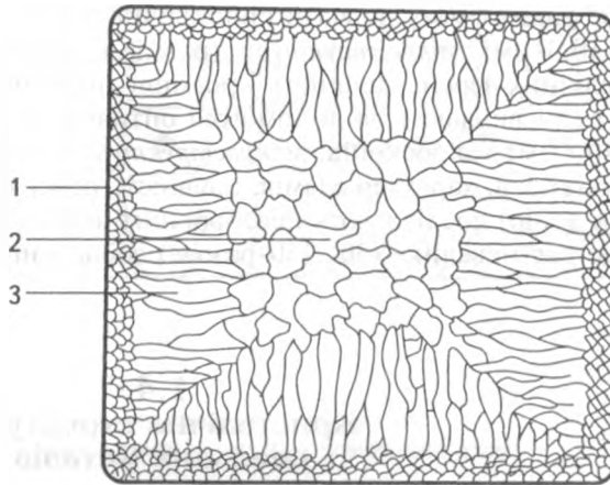
Рис. 1.6 Макроструктура зливка:
