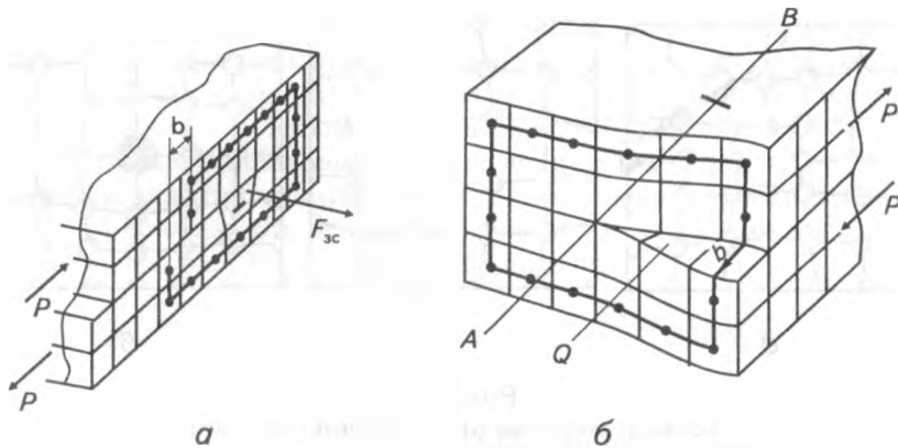
Рис. 1.8 Лінійні дефекти кристалічної решітки: a — крайова дислокація; б — гвинтова дислокація
