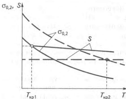
Рис. 2.18 Вплив нейтронного випромінювання на границю текучості та опір відриву за різних температур: — до дії випромінювання; - - - після
