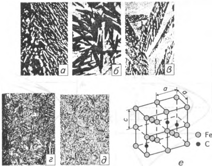
Рис. 4.10 Структури бейніту (а — верхнього; б, в — нижнього) і мартенситу (г — крупногочастого; д — дрібногочастого) та схема решітки мартенситу (е)
