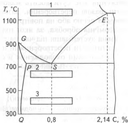
Рис. 4.22 Режими нагрівання в процесі відпалу першого роду:
