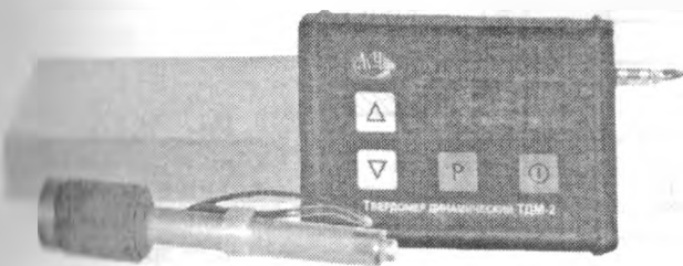
Рис. 2.15 Твердомір ТДМ-2
