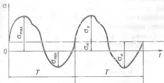
Рис. 2.9 Характеристики циклічних напружень, що змінюються за синусоїдним законом
