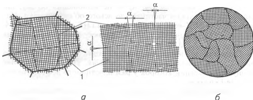
Рис. 1.4 Форми кристалічних утворень:
