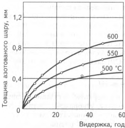
Рис. 4.33 Вплив температури й видержки на товщину азотованого шару
