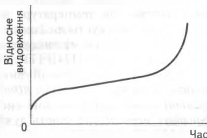
Рис. 5.7 Типова крива повзучості
