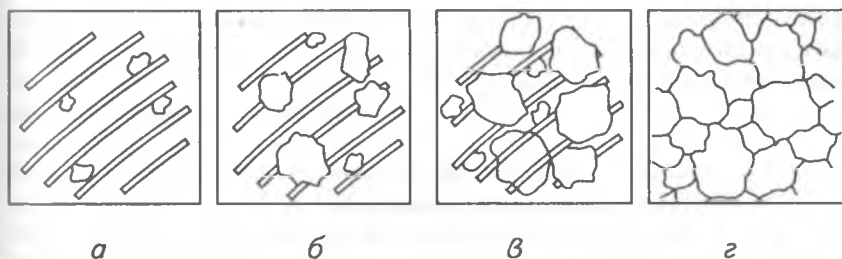
Рис. 4.2 Послідовність перекристалізації перліту в аустеніт
