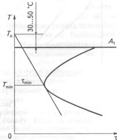
Рис. 4.12 Схема для визначення v_{кр} за діаграмою ізотермічних перетворень
