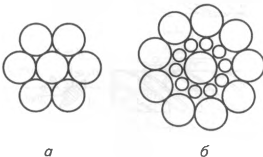
Рис. 5.3 Поперечні перерізи арматурних канатів: a — К7; б — К19
