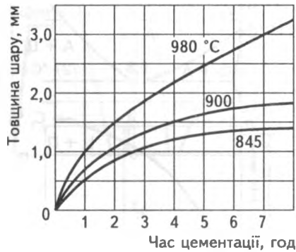
Рис. 4.30 Температурна залежність середньої тривалості й глибини цементації
