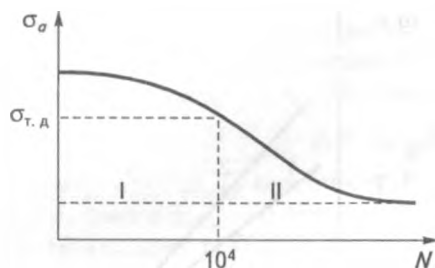
Рис. 2.11 Повна діаграма втомленості: I, II — зони відповідно мало- й багаточислової втомленості
