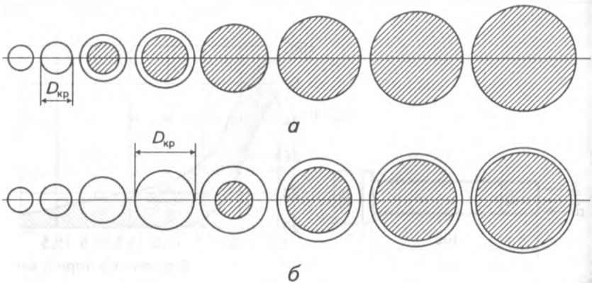
Рис. 4.19 Прогартовуваність сталевих циліндрів різного діаметра з охолодженням у воді (а) й оливі (б)
