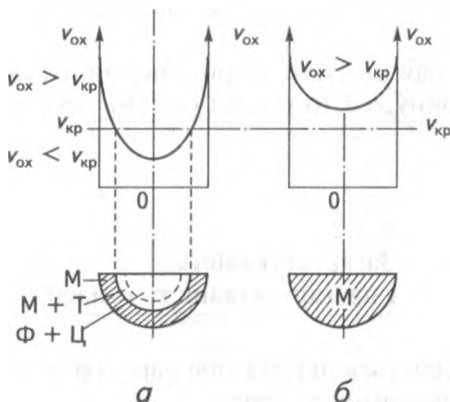
Рис. 4.16 Схема прогартовуваності циліндричної деталі: а — ненаскрізної; б — наскрізної
