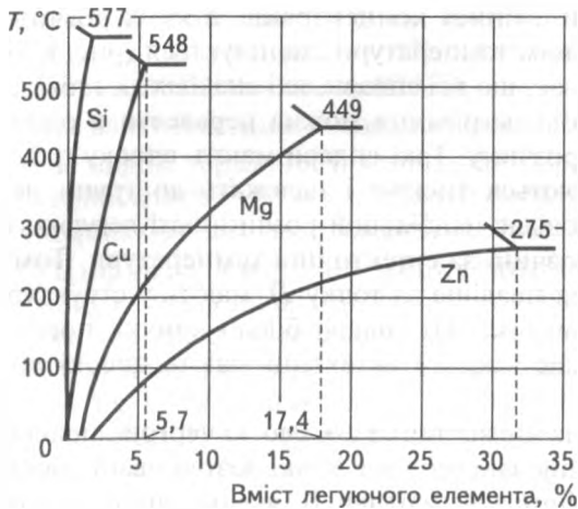
Рис. 8.4 Початкові області діаграм рівноважного стану сплавів Al із Si, Cu, Mg, Zn
