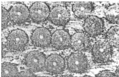
Рис. 10.1 Мікроструктура МКМ АІ—В ( V_b = 30\% ), одержаного дифузійним зварюванням
